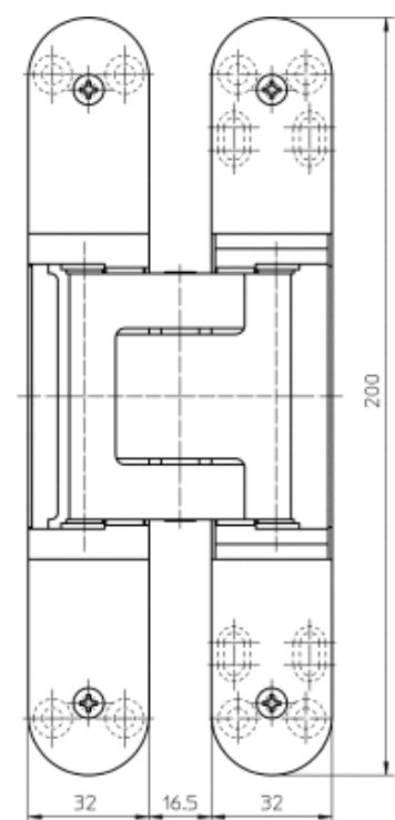
Vorderansicht
